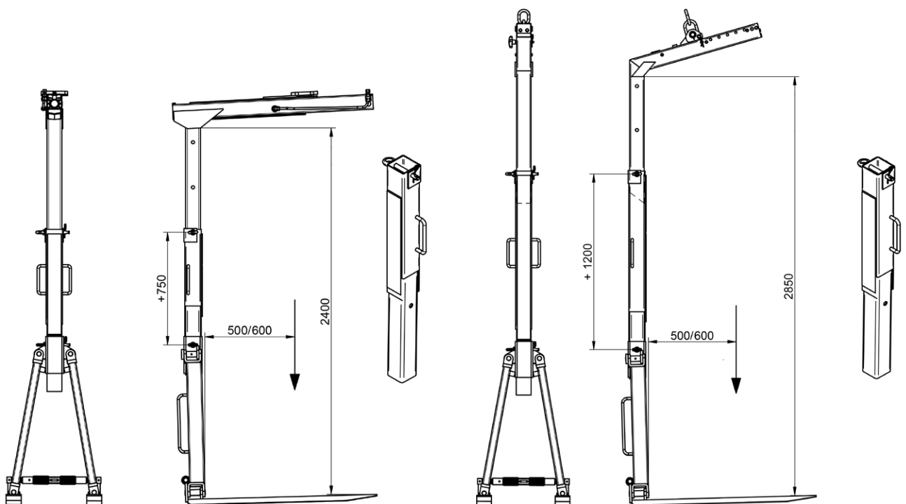
Prolunga di 750 mm su KM 401 H (senza rotatore)
